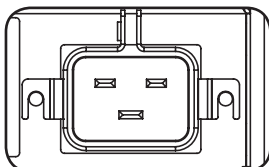
Entrada de Energía: La entrada de energía IEC-320-C20 se conecta al cable de alimentación incluido o a un cable de alimentación suministrado por el usuario. La entrada incluye un soporte para asegurar la conexión del cable.
